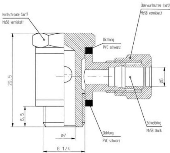
Type Nr. N 83 Art Nr. 112005
