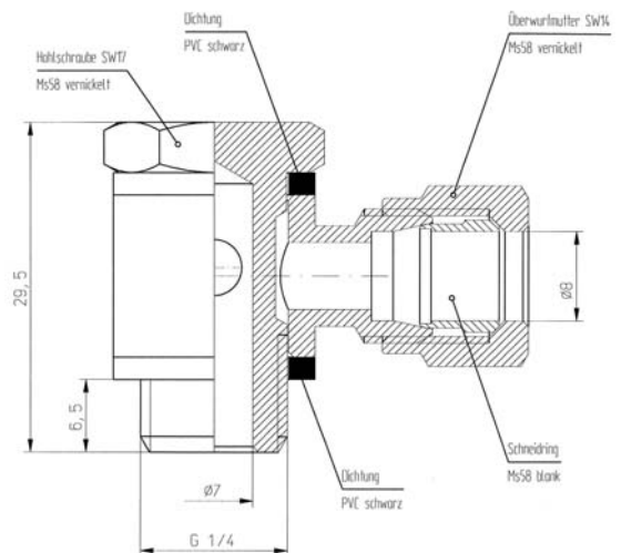
Type Nr. N 84 Art Nr. 112006
