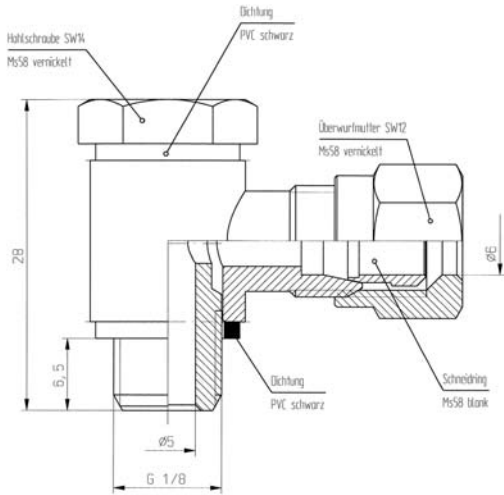
Type Nr. N 81 Art Nr. 112003
